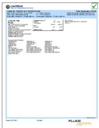
LinkWare-Bericht mit Encircled-Flux und getesteten Testreferenzleitungen
